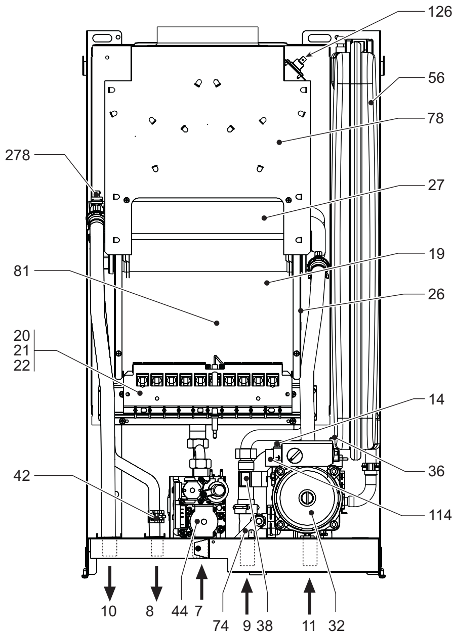
рис. 18 - Общий вид
