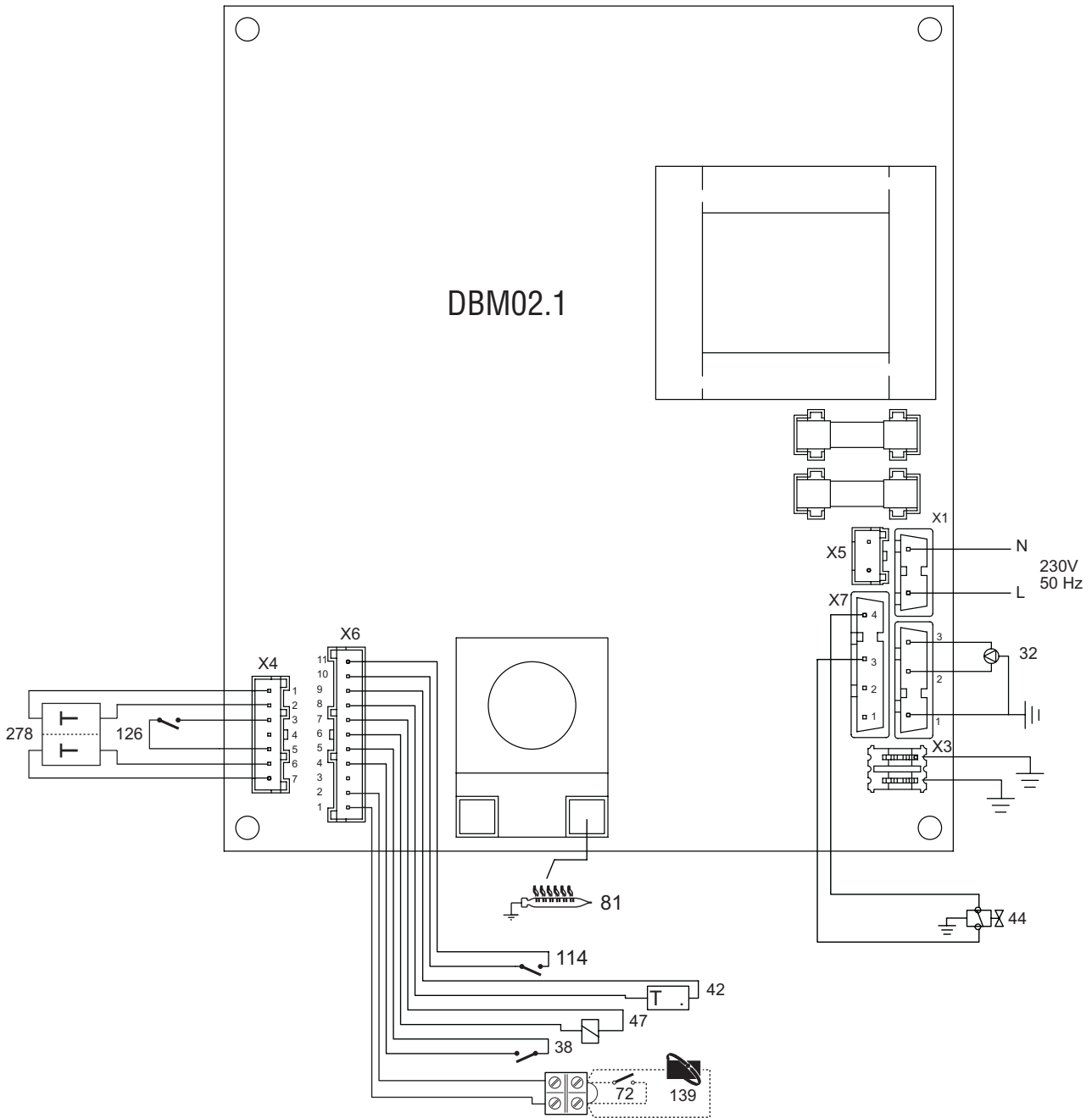
рис. 20 - Электрическая схема
